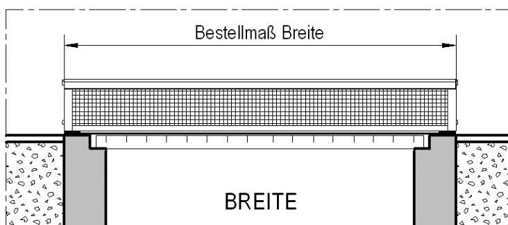
Schnittansicht Breite
