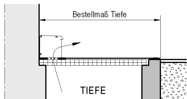
Schnittansicht Tiefe
